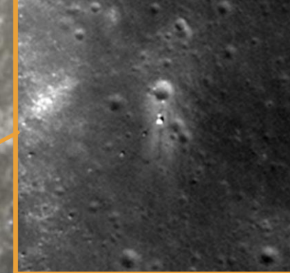
Chang'e 3
